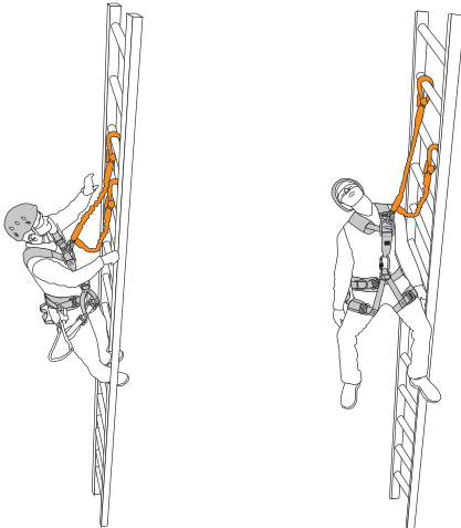
H.1 - Göğüsten Kullanım A Ankrāj Noktası (Şekil - 1.1) Use of Sternal A Attachment Point (Figure -1.1)
