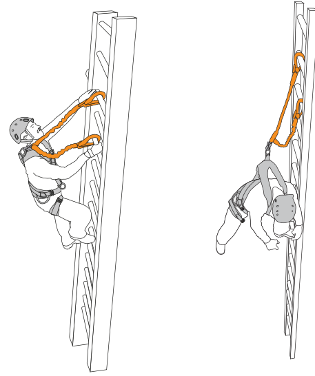
H.2 - Sırttan Kullanım A Ankrāj Noktası (Şekil - 1.2) Use of Dorsal A Attachment Point (Figure -1.2)
